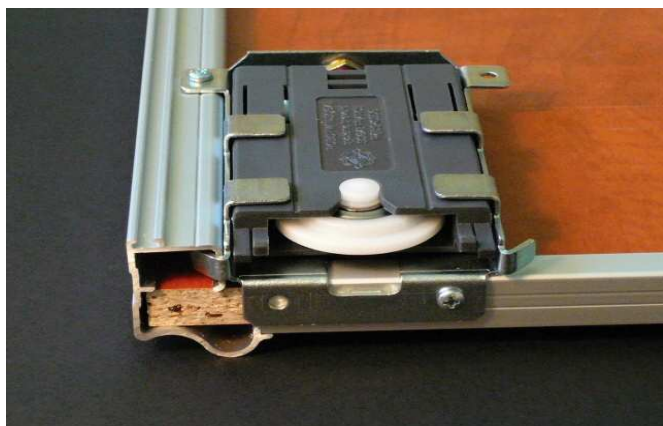
UCHYCENÍ SPODNÍHO KOLEČKA - RAIL
