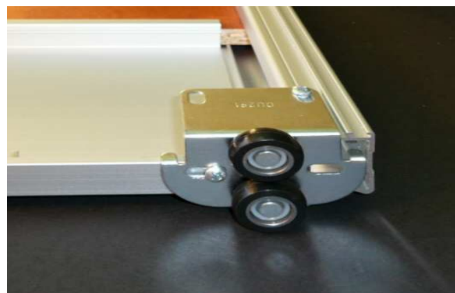
UCHYCENÍ HORNÍHO KOLEČKA - PLINTH
