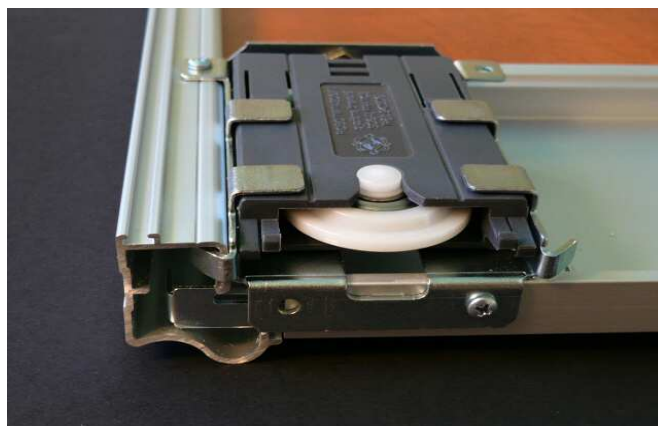
UCHYCENÍ SPODNÍHO KOLEČKA - PLINTH
