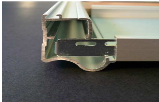
SVISLÁ LIŠTA MADONA, VODROVNÁ LIŠTA PLINTH
