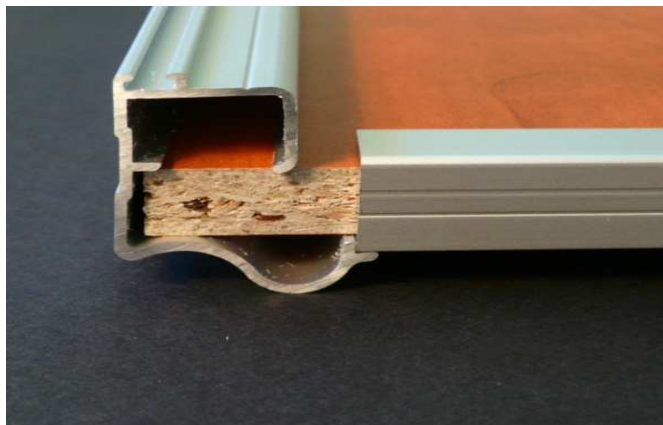
SVISLÁ LIŠTA MADONA, VODROVNÁ LIŠTA RAIL
